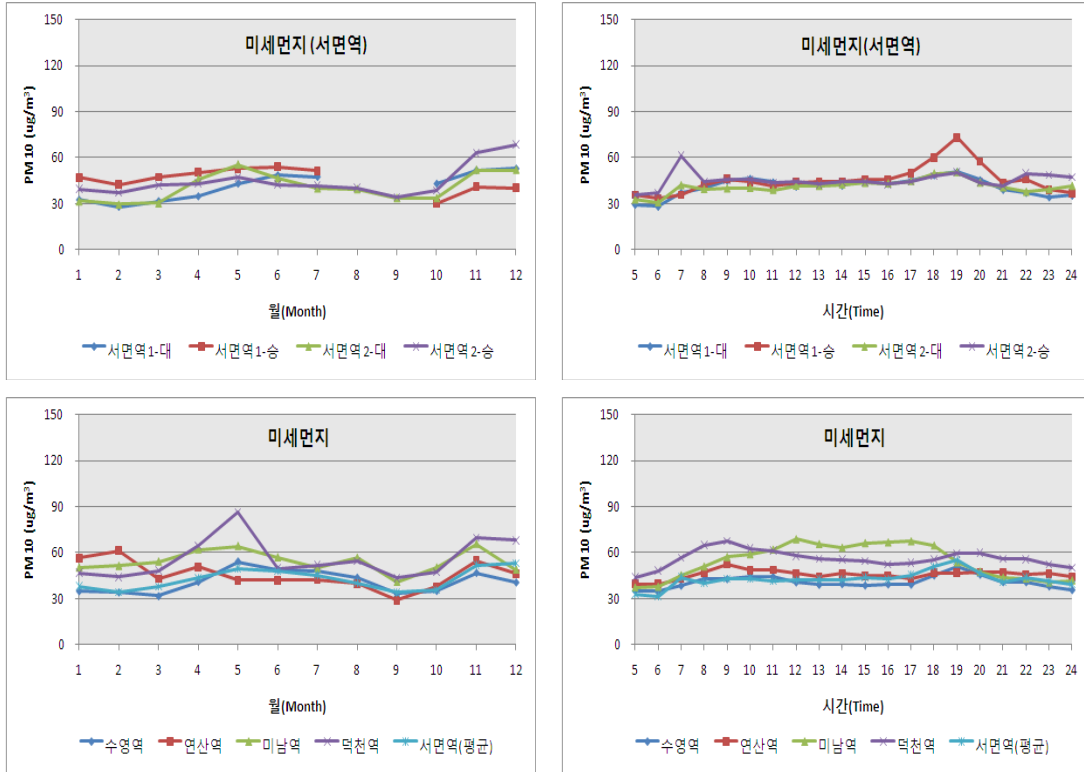
그림 1. 측정소별 미세먼지(PM10)의 일별 및 시간별 농도 변화
