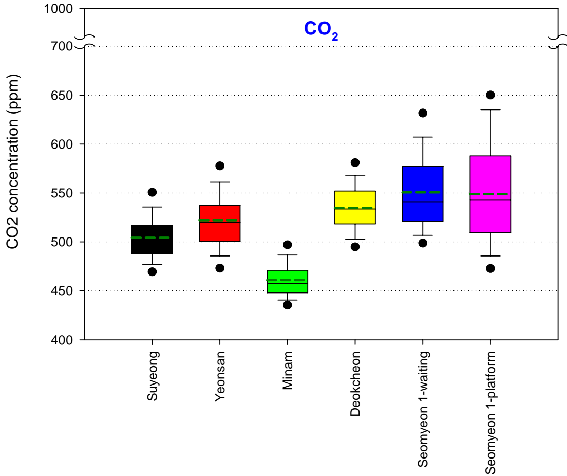
그림 9. 측정소별 이산화탄소(CO 2 )의 일평균 농도분포
