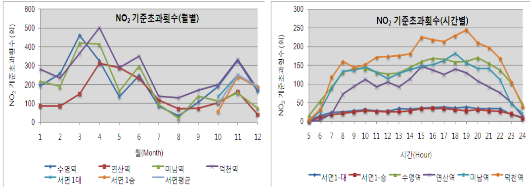
그림 14. NO 2 의 월별 및 시간별 권고기준 초과현황
