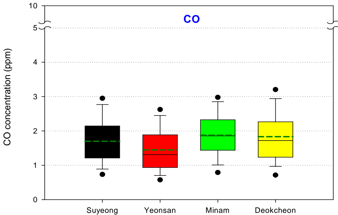
그림 8. 측정소별 일산화탄소(CO)의 일평균 농도분포
