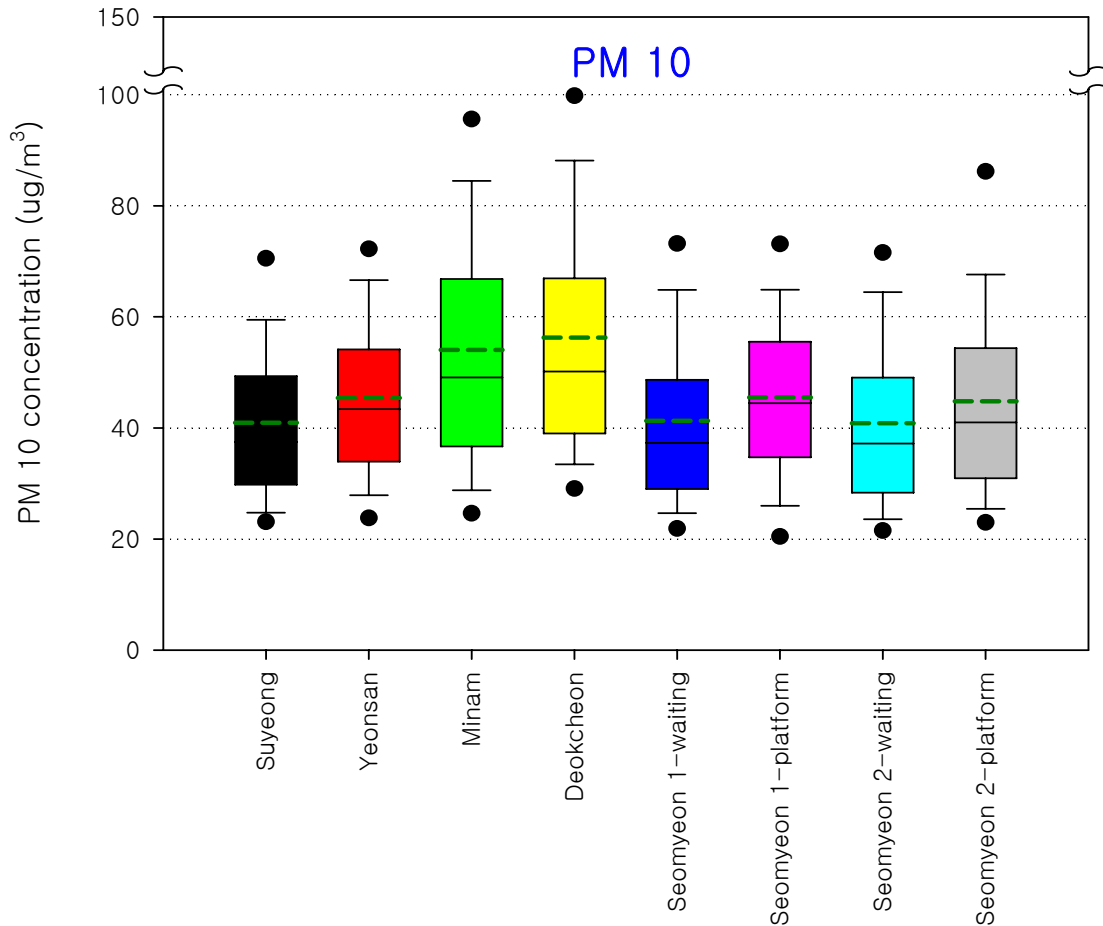
그림 7. 측정소별 미세먼지(PM10)의 일평균 농도분포
