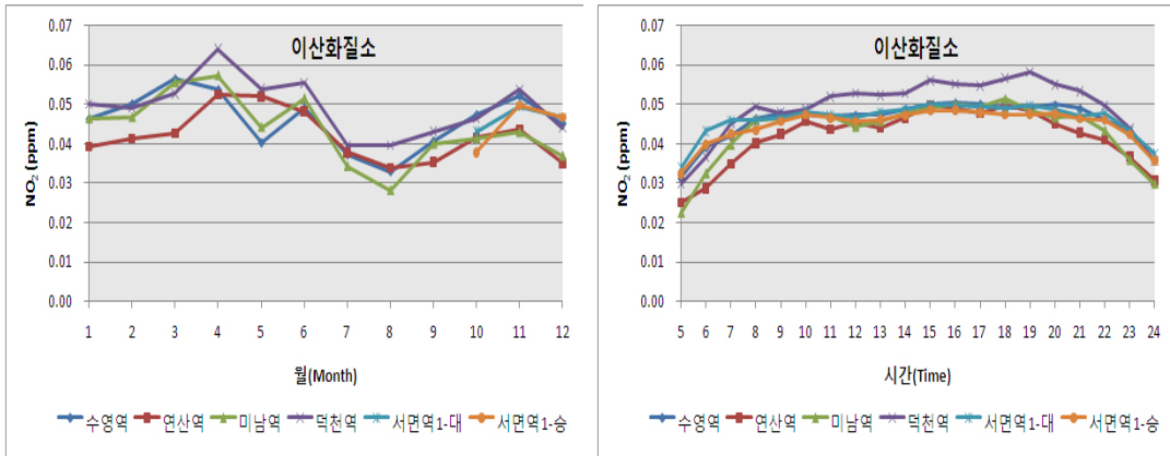
그림 5. 측정소별 이산화질소(NO2)의 일별 및 시간별 농도 변화
