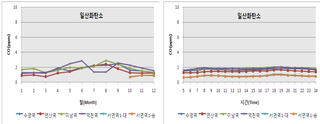
그림 3. 측정소별 일산화탄소(CO)의 일별 및 시간별 농도 변화
