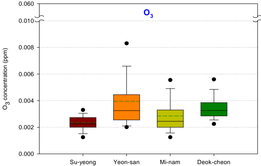
그림 11. 측정소별 오존(O3)의 일평균 농도분포
