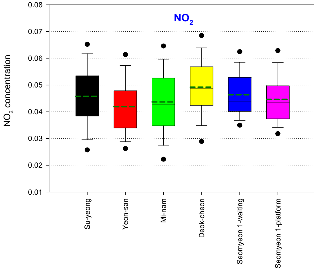
그림 10. 측정소별 이산화질소(NO 2 )의 일평균 농도분포
