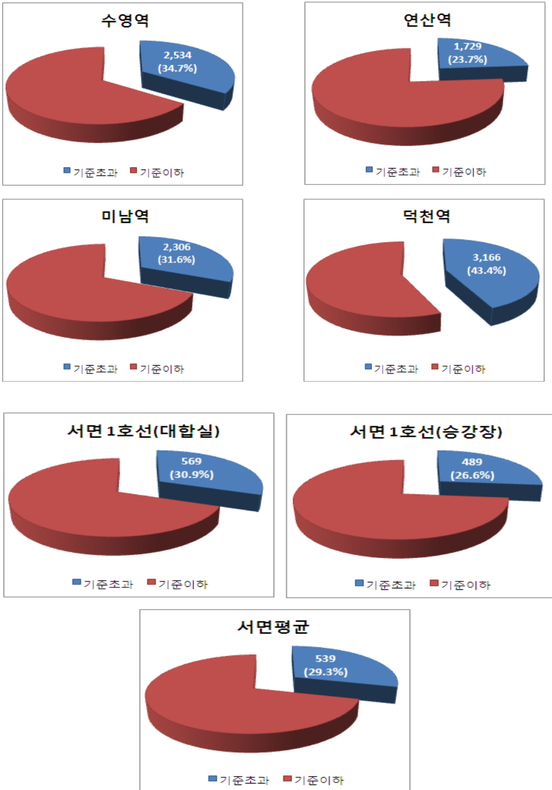
그림 13. NO 2 의 권고기준 초과현황
