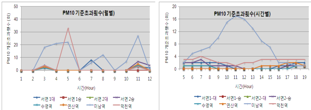
그림 12. PM10의 월별 및 시간별 유지기준 초과현황
